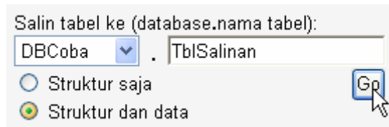
Gambar 4.11 Menyalin tabel
